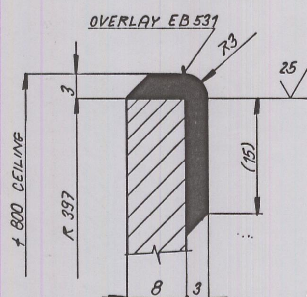
D (2:1)
