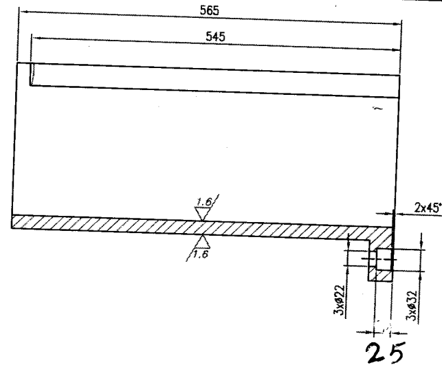
SEC A-A
