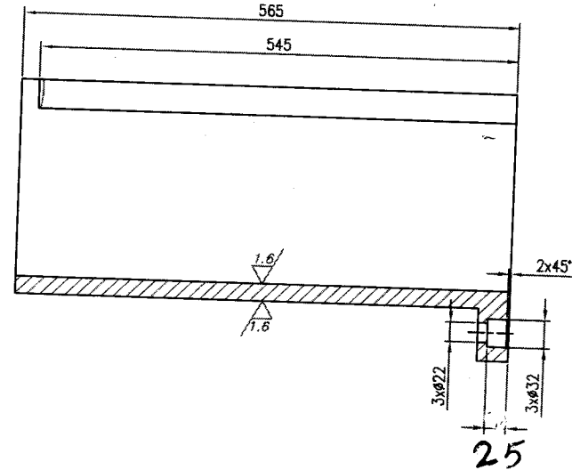
SEC A-A
